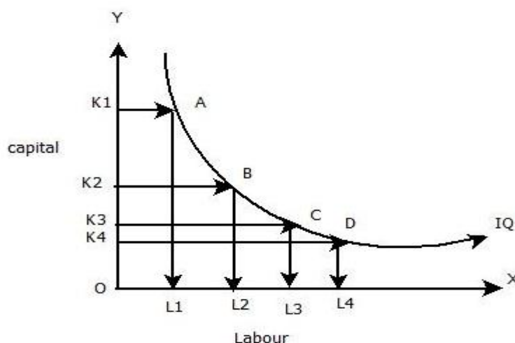
Fig. 3.1.3 Isoquant
