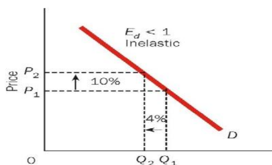
Fig. 2.1.11.5 Inelastic
